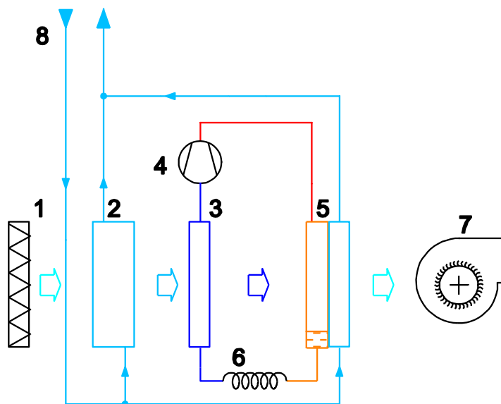
Fig. 1 Schema del deumidificatore DMC
